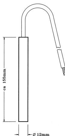
Fig. 1 Dimensions (mm)
