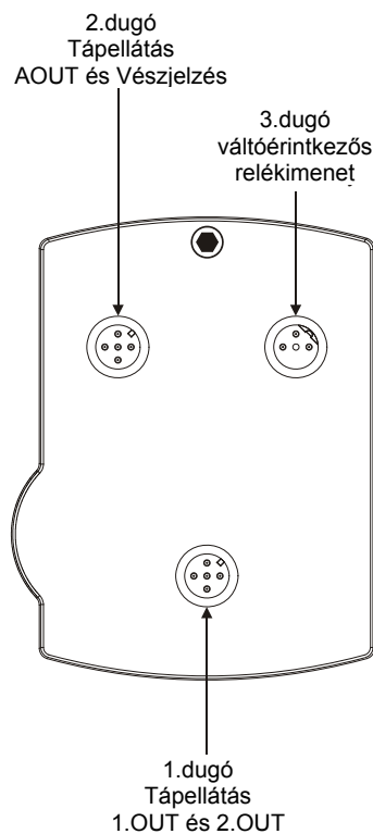
Fig. 2. PST...-R sorozat házának hátlapja
