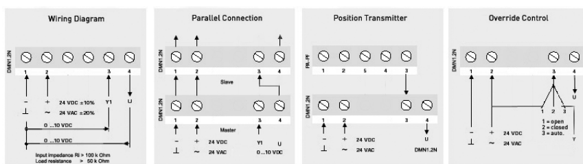
Villamos bekötés
