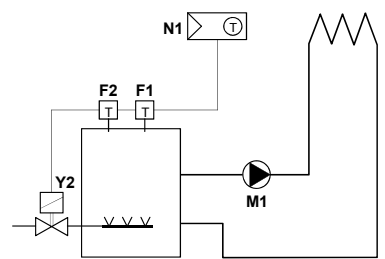
Szobatermosztát álló gázkazán direkt szabályozásával
